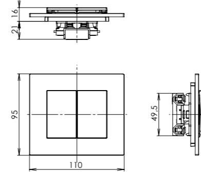
spínač s dvojitým krytem
