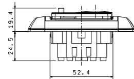
analogový termostat OREG/EBERLE DSE 2T/3T
