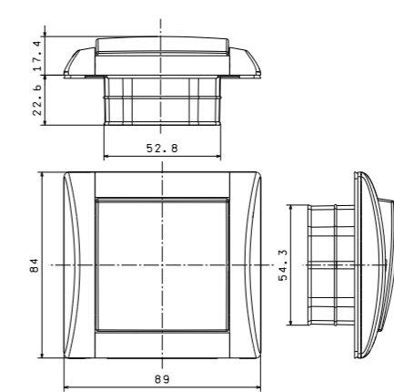
spínač IP 44 s jednoduchým krytem
