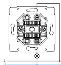
spínač řazení 1 (jednopolový vypínač)
