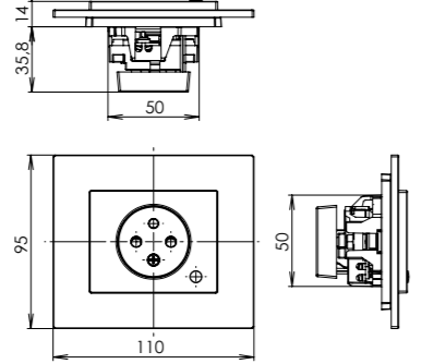
zásuvka jednonásobná s clonkou a přepětovou ochranou
