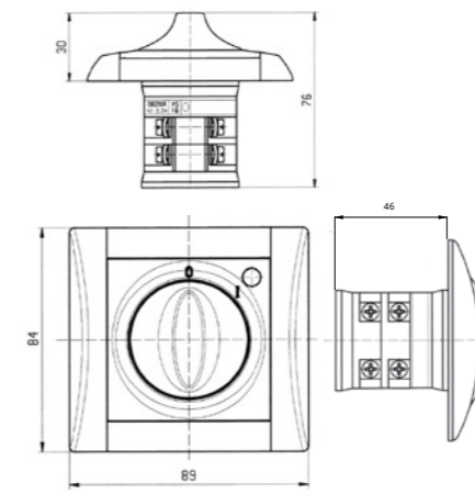
sporákový spínač otočný
