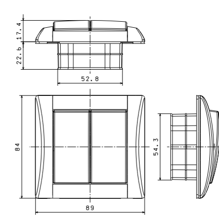
spínač IP 44 s dvojitým krytem
