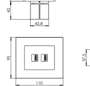
zásuvka modulová USB nabíječka
