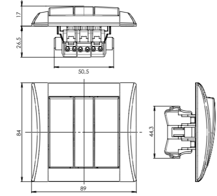
spínač s trojitým krytem
