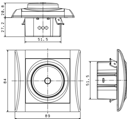
stmívač otočný s tlačítkovým spínačem PUSH-PULL a funkcí řazení č. 6
