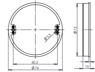
vymežovací kroužek VK1
