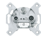
zásuvka TV+SAT+SAT průběžná, útlum 10 dB, 300 mA, 24 V DC pro koaxiální kabely průměru 4,5–8,3 mm typové označení na výrobku: ZAR-SAT 10/P3
