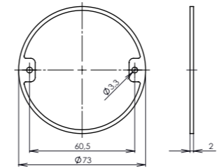
vymežovací kroužek VK2
